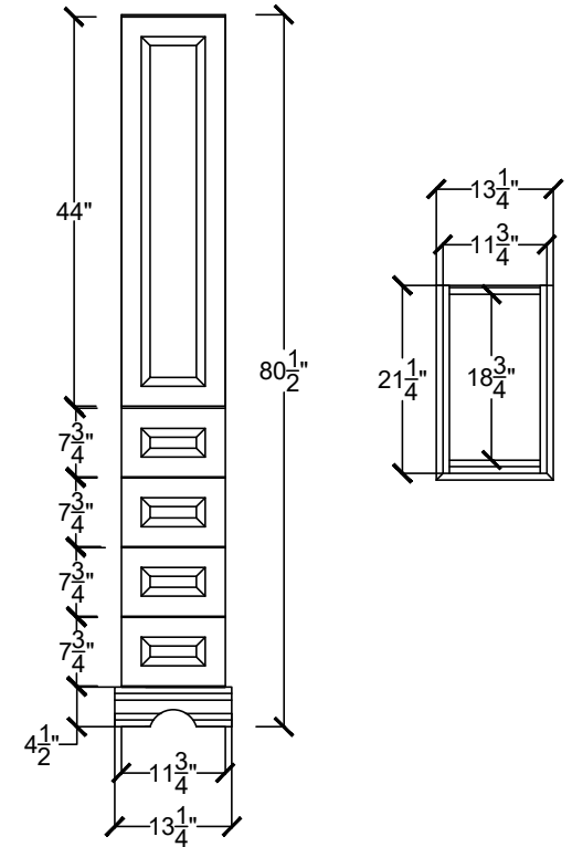
H-ARTTC 1222-4D- _____ - _____ - _____
