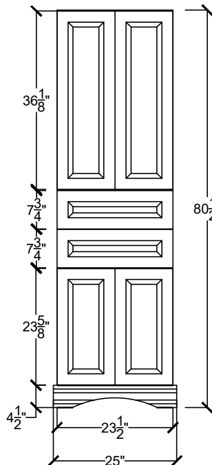
H-ARTTC 2422-2D-____-____-____
