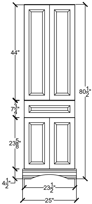
H-ARTTC 2422-1D-____-____-____
